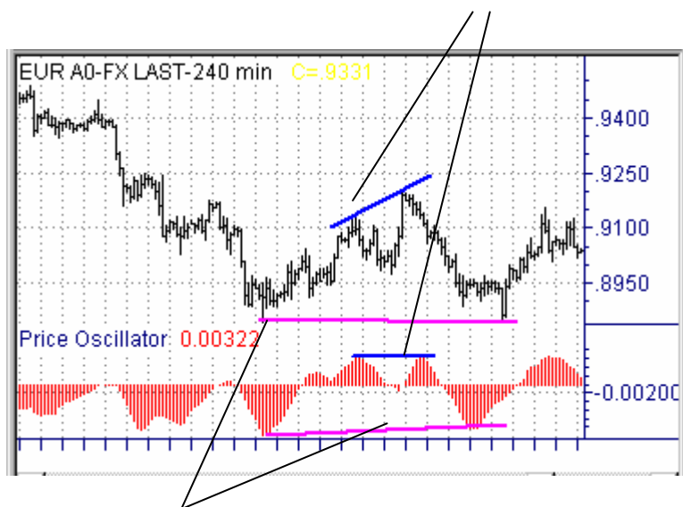
Пример дивергенции
