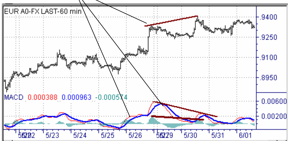
Пример дивергенции
